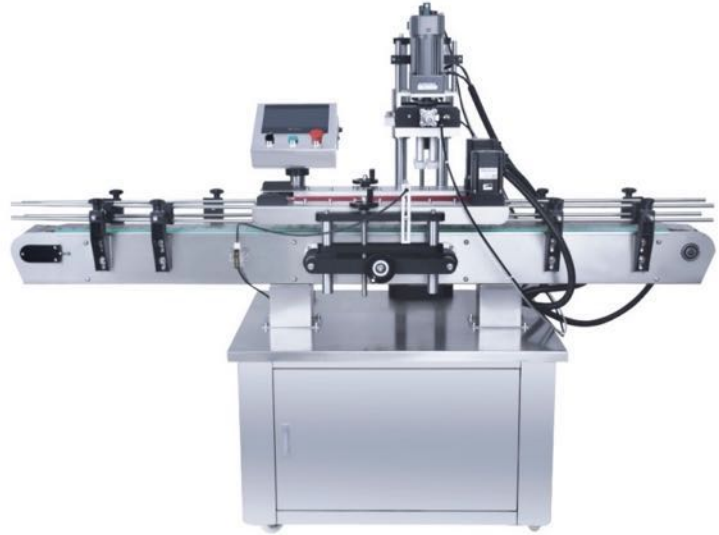
全自动搓盖机 AUTOMATIC CAPPING MACHINE
